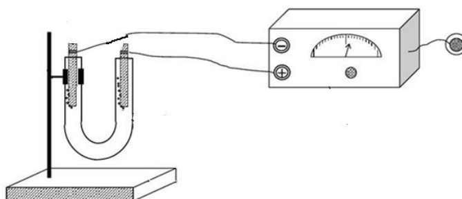
Рис. 1. Схема установки для электролиза растворов
